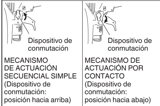
Dispositivo de conmutación para la operación de clavado
